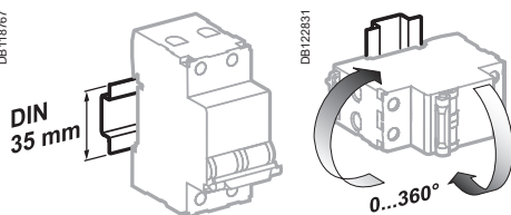
Clip on DIN rail 35 mm (1.38 in)
