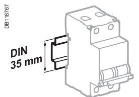
Clip on DIN rail 35 mm (1.38 in)
